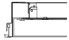
TB9 - t-bar 9/16"
