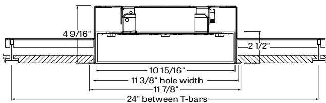
POSQR- TB9 - t-bar 9/16"
