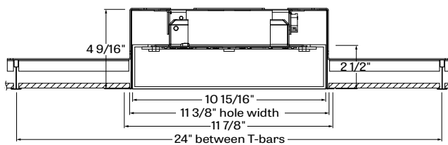
POSQR- TB9 - t-bar 9/16"
